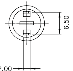
Solder Lug
